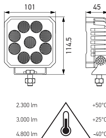
Rysunek wymiarowy
