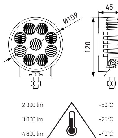
Rysunek wymiarowy
